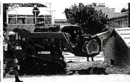
多機能重機車の遠隔操作による倒木の撤去
